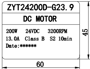
电机铭牌
