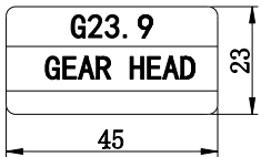
减速器铭牌
